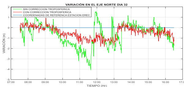
Fig. 8. Variación del Error de Retardo Troposférico en el Eje Norte correspondiente al día 32.
