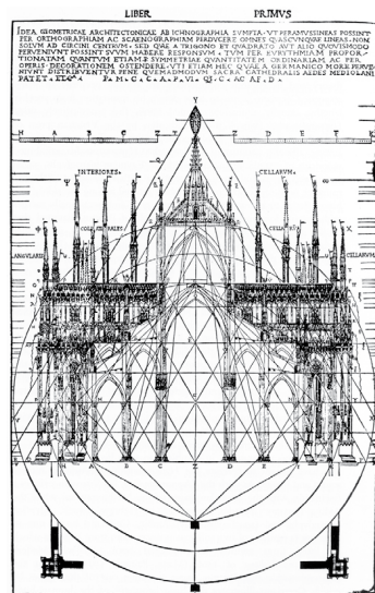
Fig. 3. Sistema proporcional por triangulación: ad triangulum. Idea geometricae architectonicae: Milan Cathedral (Cesariano) [17, p. 3].
