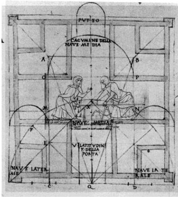
Fig. 2. Sistema proporcional con el cuadrado: ad quadratum. Chiesa maggior under construction ad quadratum (Filarete, Francesco di Giorgio, Prudence) [17, p. 3].
